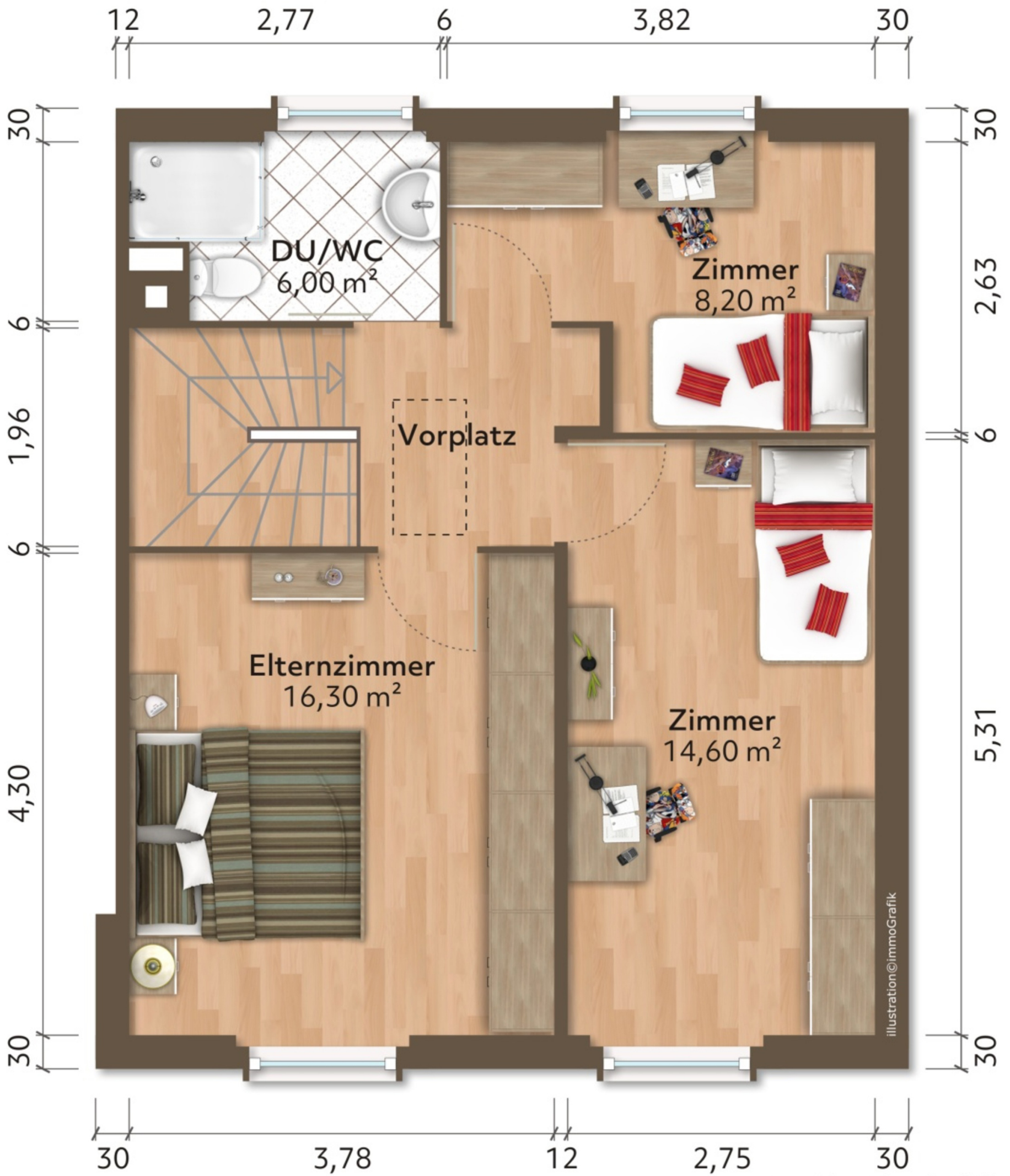
Exposéplan, nicht maßstäblich
